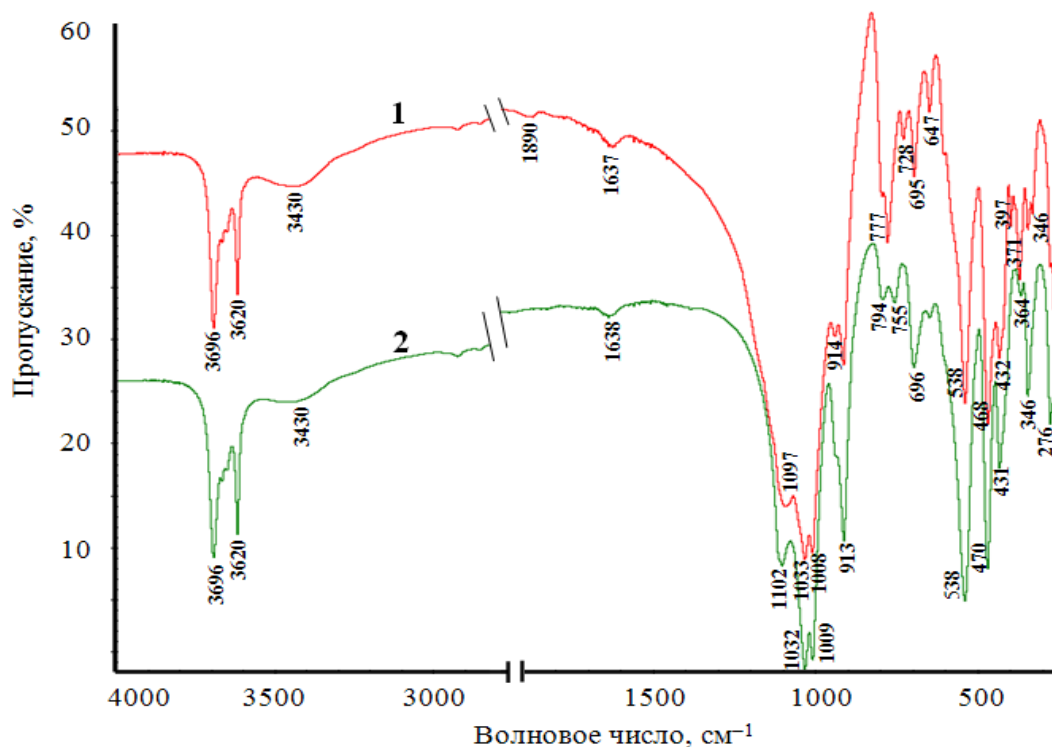
Рис. 2 – Инфракрасные спектры поглощения каолина месторождения «Дедовка»: 1 – природный; 2 – обогащенный
