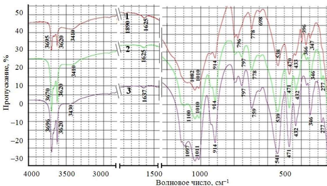
Рис. 1 – Инфракрасные спектры поглощения каолинов месторождений: 1 – «Ситница» (природный); 2 – «Ситница» (обогащенный); 3 – Просьяновское
