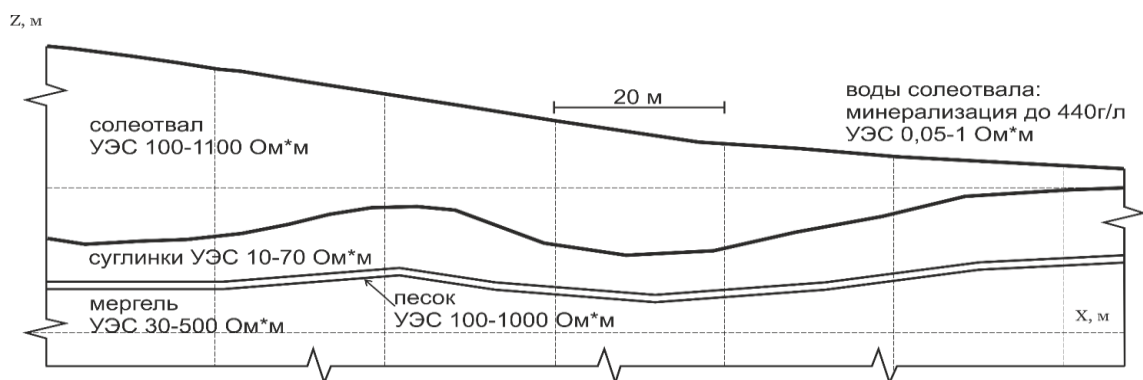
Рис. 2 – Разрез по геолого-геофизической модели участка исследований
