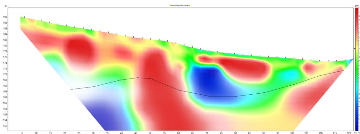
Рис. 3 – Разрез УЭС по профилю 4, полученный в результате 2D-инверсии данных электротомографии
