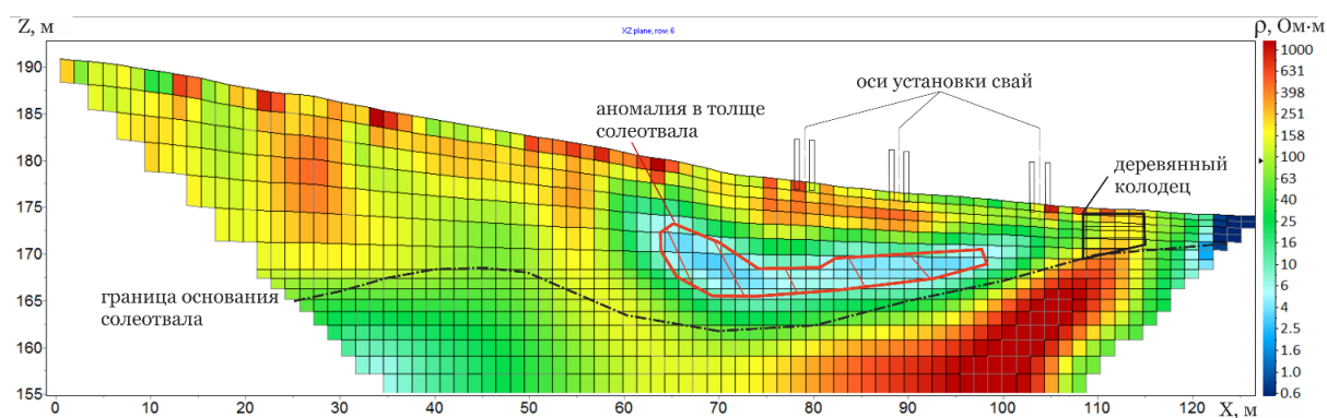
Рис. 5 – Блочная модель УЭС по профилю 4 с зонами разуплотнения
